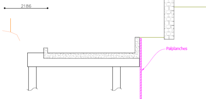
Coupe 1-1
