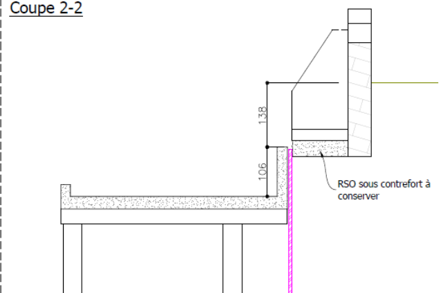
Coupe 2-2
